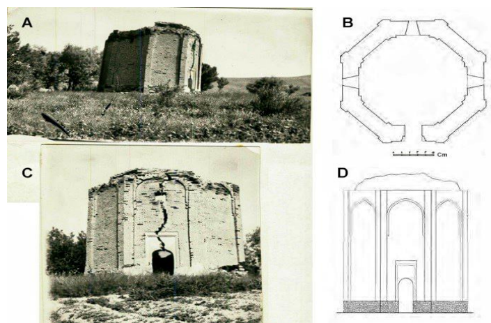
تصویر ۲. نما، پلان و مقطع برج اشقون بابا روستای علیشه دهستان سیاه منصور (آرشیو میراث فرهنگی کردستان، ۱۳۵۲)
