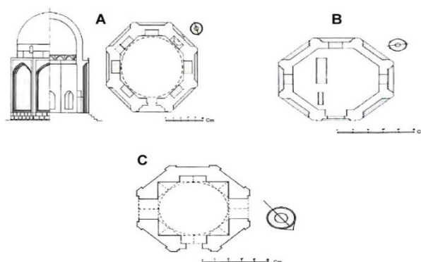
تصویر ۲. نما، پلان و مقطع برج اشقون بابا روستای علیشه دهستان سیاه منصور (آرشیو میراث فرهنگی کردستان، ۱۳۵۲)
