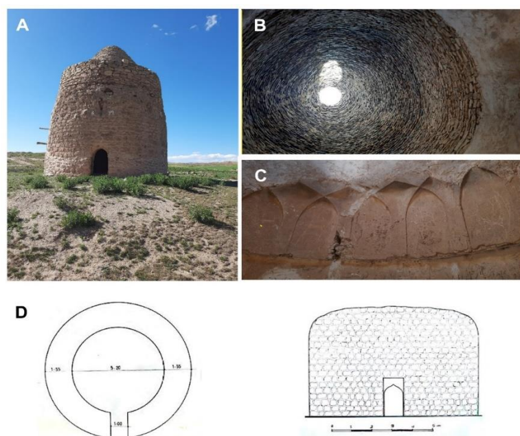
تصویر ۴. پلان، نما و مقطع برج ینگى ارخ (آرشیو میراث فرهنگی کردستان، ۱۳۵۲ و ۱۳۶۳)
