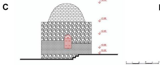
تصویر ۷. پلان، نما و مقطع برج شمالی قمچقای قبل و بعد از مرمت
