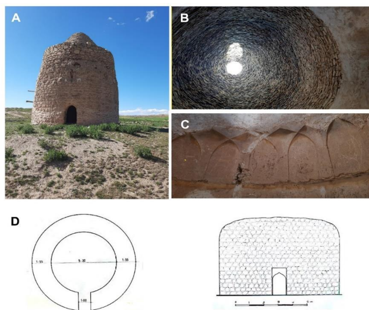
تصویر ۴. پلان، نما و مقطع برج ینگى ارخ (آرشیو میراث فرهنگی کردستان، ۱۳۵۲ و ۱۳۶۳)
